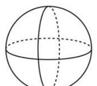
Kugel
