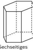
Sechseitiges Prisma
