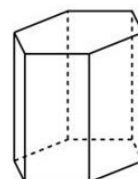
Sechseitiges Prisma
