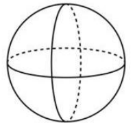
Kugel
