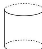
Zylinder
