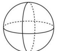
Kugel
