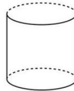
Zylinder
