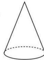
Kegel
