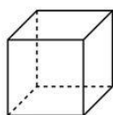
Würfel
